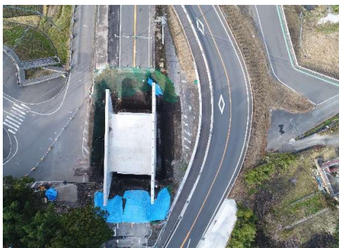
着工前 (旧国道函渠部) 上空より望む
